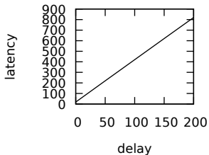
/deposit
